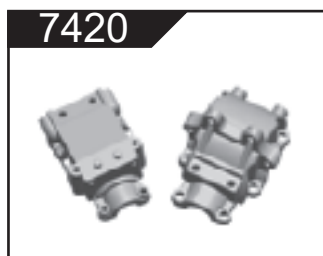
7420 Differtentialgehäuse vorne oder hinten
